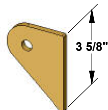
12281-5 1/4" MAT
