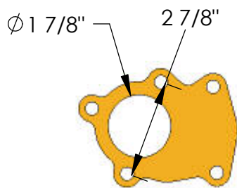
12201 GT 28 FLANGE
