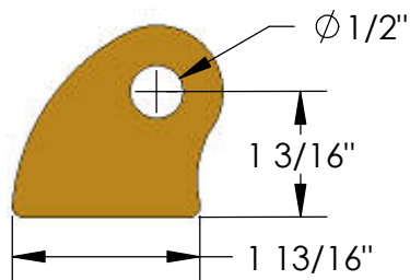
12274 PARACHUTE TAB
