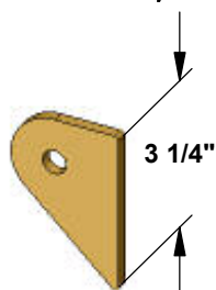
12281-4 1/4" MAT
