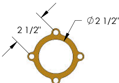
12198 TURBO FLANGE
