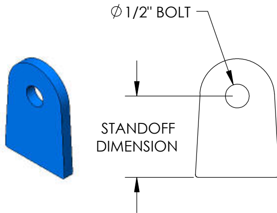
FLAT TAB
