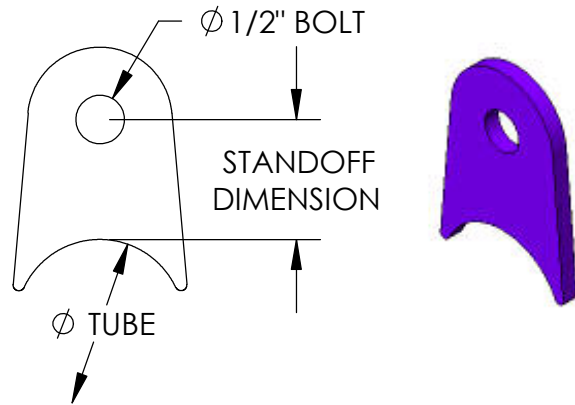
RADIUS TAB
