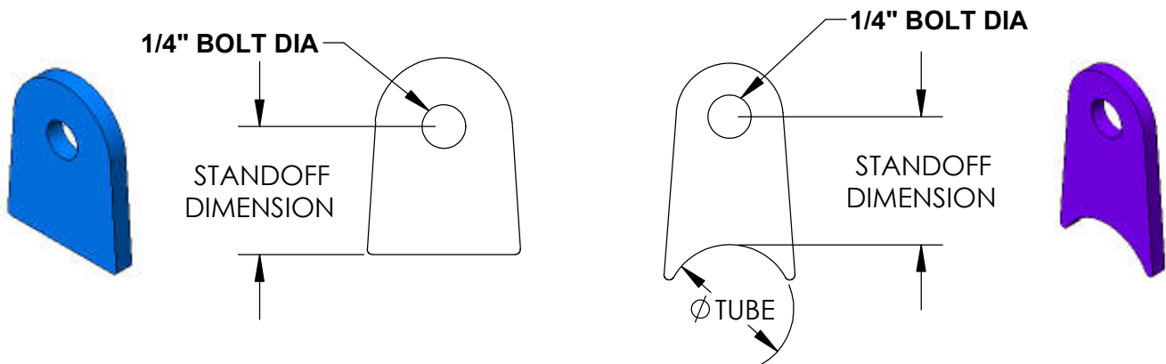
FLAT TAB
